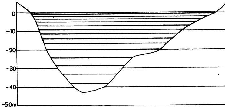
Попречни профил кроз дно Верига.
